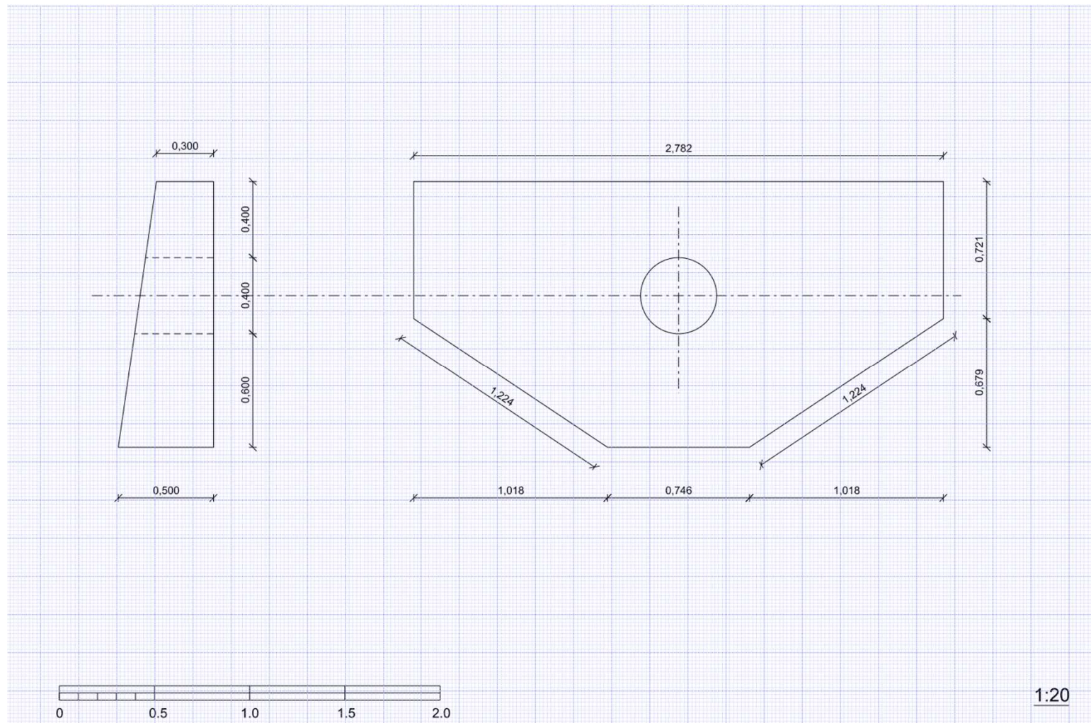
Indløbsbygværk (type VD 26611, Ø400mm)
